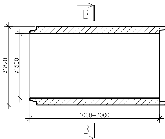
PRZEKRÓJ A-A
