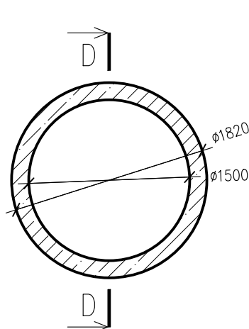
PRZEKRÓJ C-C
